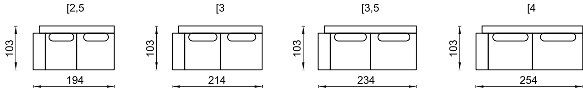
END ELEMENT FIN ÉLÉMENT
