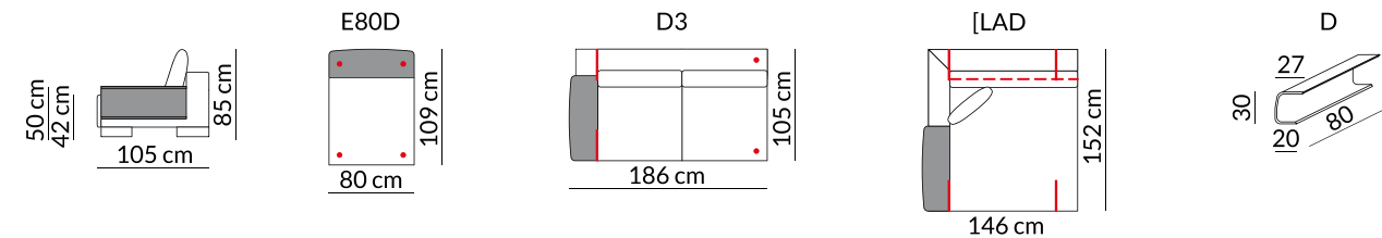
ELEMENTS THAT CAN BE ORDERED WITH A WOODEN ARMREST ÉLÉMENTS POUVANT ÊTRE COMMANDÉS AVEC UN ACCOUDOIR EN BOIS
