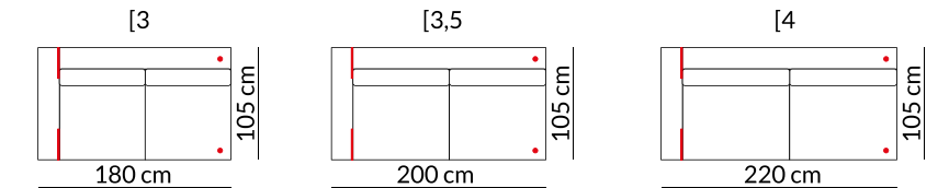
END ELEMENT FIN ÉLÉMENT
