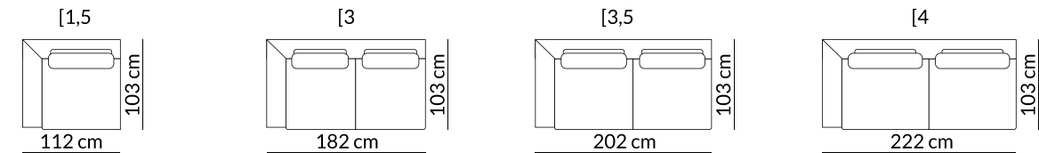
END ELEMENT FIN ÉLÉMENT
