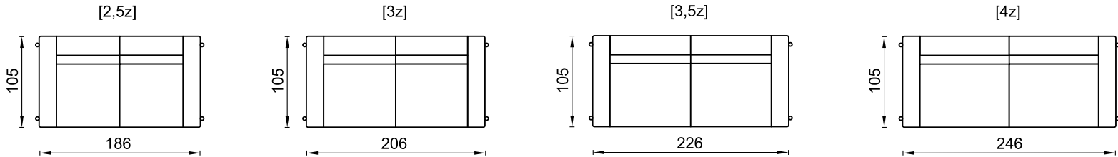
END ELEMENT FIN ÉLÉMENT
